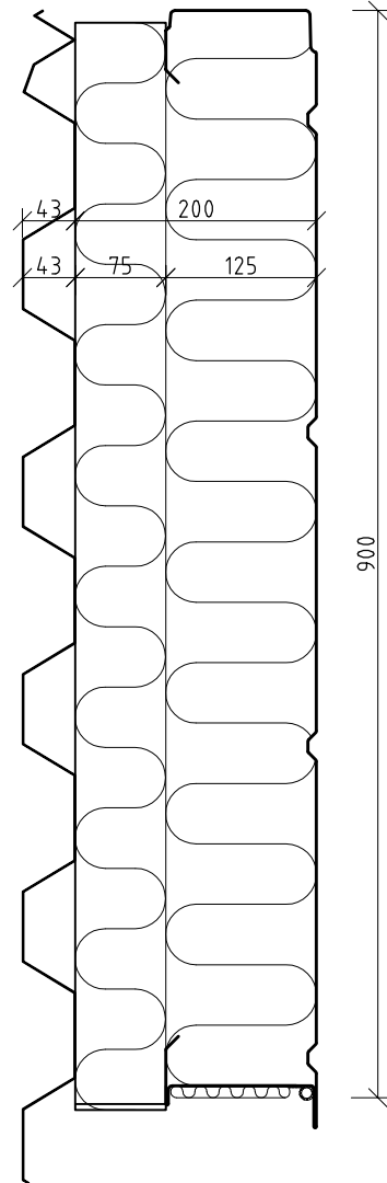
KVATRO THR43 200
