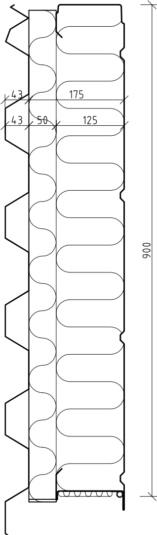
KVATRO THR43 175
